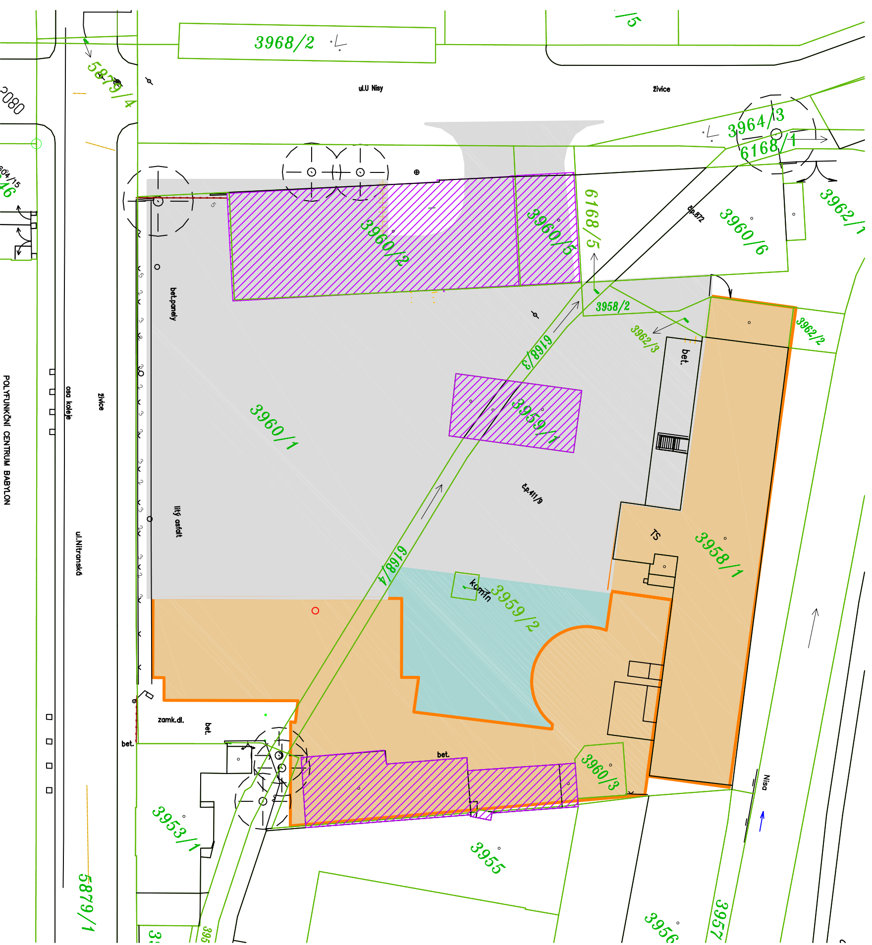
SITUACE KATASTRÁLNÍ 1:500
